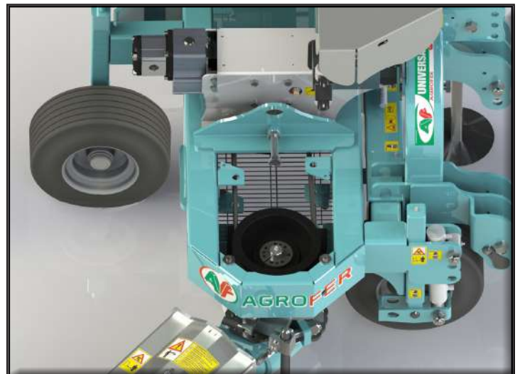
TRANSMISSION MÉCANIQUE DU DISQUE
