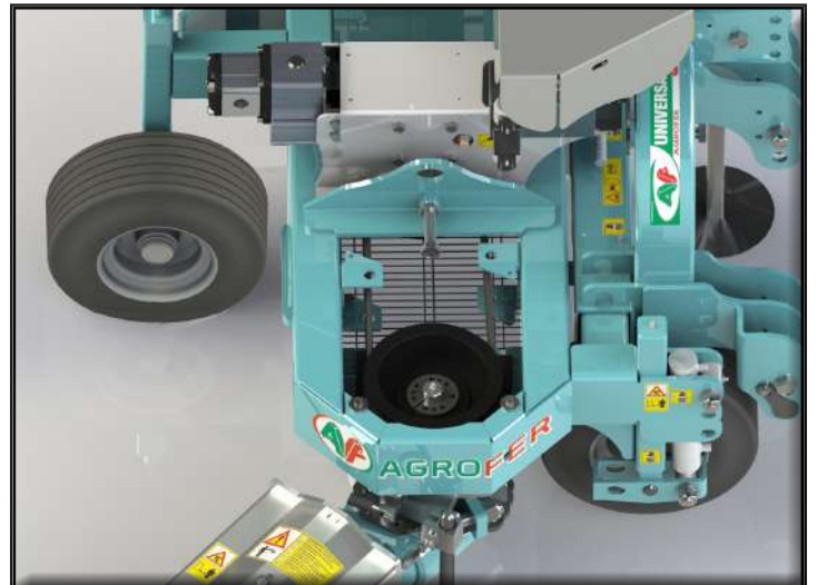
MECHANISCHER ANTRIEB DES SCHEIBENAGGREGATS
