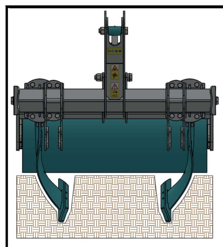
ANCRES RECOURBÉES
